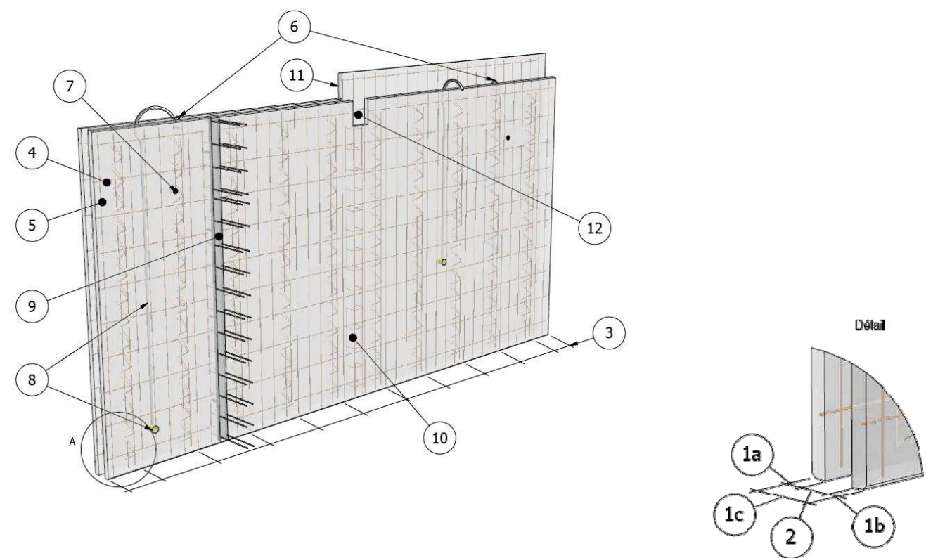
Fig 1: Vue générale d'un Prémur Rector
