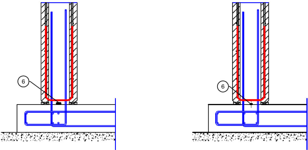
6 Joint waterstop en tôle ou joint hydrogonflant
